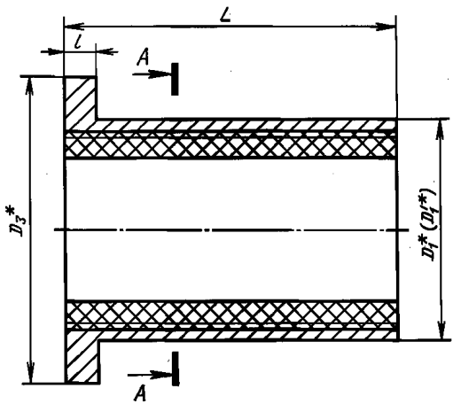
Подшипник типа II
