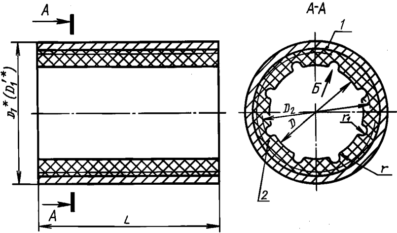
Подшипник типа I
