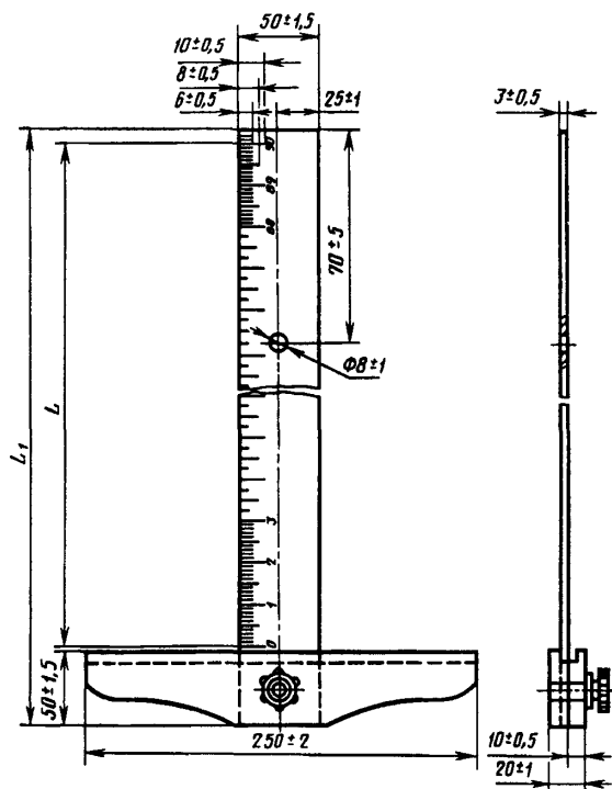
Рейсшина типа РДД
