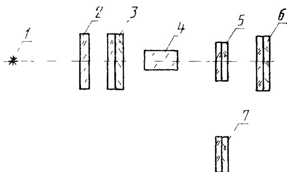
1 — источник света, 2 — матовое стекло, 3 — поляризатор, 4 — испытуемый образец, 5 — фазовая пластинка \lambda/4 , 6 — анализатор, 7 — фазовая пластинка \lambda/4
