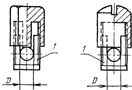
1 — неподвижная деталь; D — место расположения проводника*
