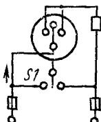
Выключатель по схеме 6/2
