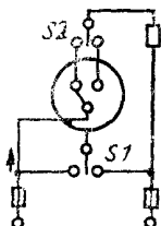
Выключатель по схеме 6
