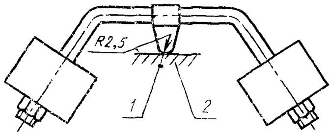
1 — сфера; 2 — испытательный образец
