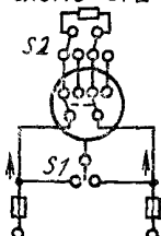
Выключатель по схеме 6/2
