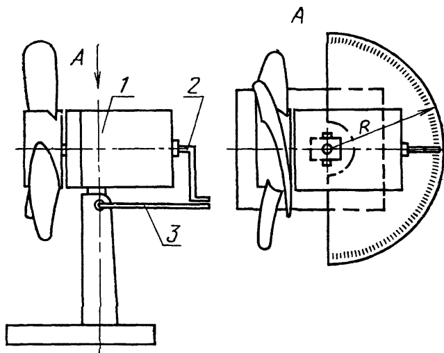
1—корпус вентилятора; 2—стрелка-указатель; 3—измерительная шкала
