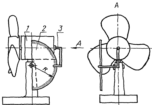
1—корпус вентилятора; 2—измерительная шкала; 3—стрелка-указатель
