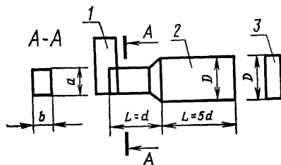
1—вентилятор; 2—переходной цилиндр; 3—анемометр
