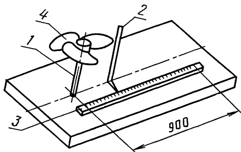
1—вал; 2—указатель; 3—шкала; 4—крыльчатка
