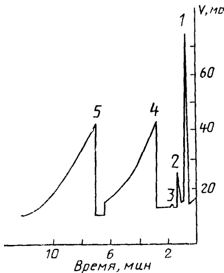
Типовая хроматограмма анализа окиси этилена
