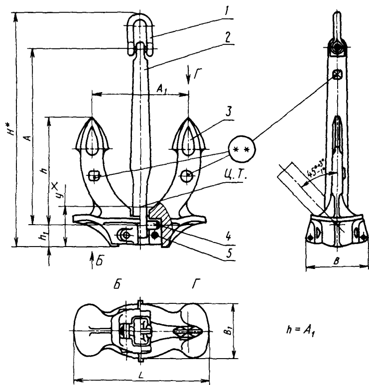
Якорь Холла с веретеном круглого сечения
