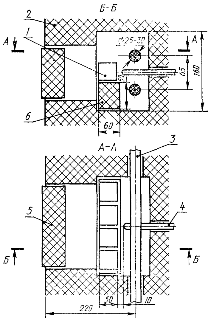
1 — образец; 2 — футеровка печи; 3 — карбидкремни- вый электронагреватель; 4 — термоэлектрический пре- образователь; 5 — дверца печи; 6 — подставка
