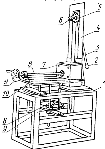
Установка для испытания моноблоков на ударную прочность
