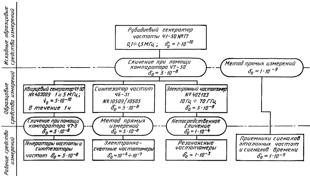
Поверочная схема для средств измерений времени и частоты
