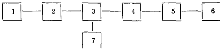
1—измерительный генератор; 2—фильтр; 3, 5—коаксиальные соединители, 4—образцовый делитель напряжения, 6—поверяемый вольтметр, 7—образцовый вольтметр
