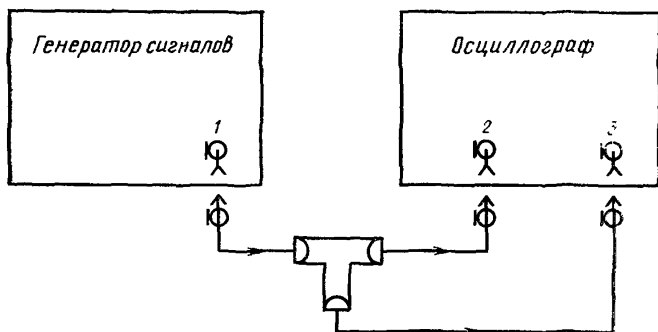
1—выход сигнала, 2—вход канала Y; 3—вход синхронизирующего сигнала
