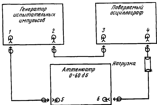
1—выход основных импульсов; 2—выход синхронизирующих импульсов, 3—вход синхронизации; 4—вход усилителя \mathcal{U} ; 5—вход аттенюатора; 6—выход аттенюатора
