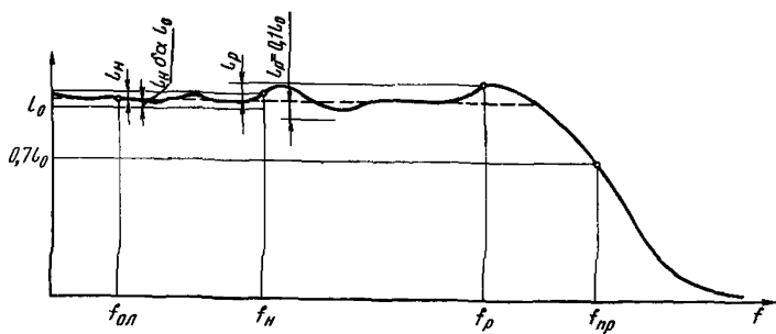
f_{оп} — опорная частота; f_н — нормальный диапазон; f_p — расширенный диапазон; f_{нр} — верхняя граница полосы пропускания; l_0 — значение АЧХ на опорной частоте; l'_н — абсолютное значение неравномерности в нормальном диапазоне; l'_р — абсолютное значение неравномерности в расширенном диапазоне; \delta_\alpha — относительная погрешность коэффициента отклонения
