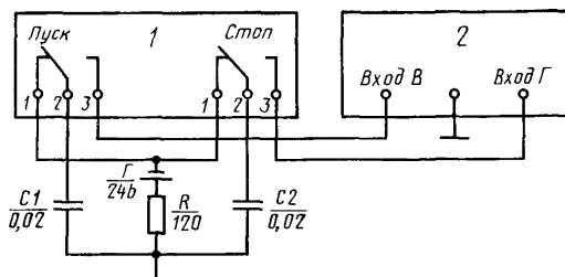
1—поверяемый прибор, 2—электронно счетный частотомер, C1 и C2—электрические постоянные конденсаторы R—постоянный резистор, Г—источник постоянного тока
