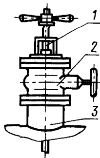
1 — сальниковый ввод; 2 — задвижка (затвор); 3 — патрубок; 4 — шлюзовая камера
