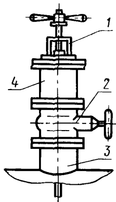
1 — сальниковый ввод; 2 — задвижка (затвор); 3 — патрубок; 4 — шлюзовая камера
