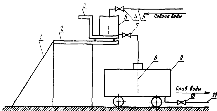
1—лестница; 2—эстакада; 3—весы; 4—запорный кран; 5—наливной трубопровод; 6—вспомогательная тара; 7—сливной кран; 8—сливной шланг; 9—ТМ; 10—сливной кран ТМ; 11—сливной трубопровод
