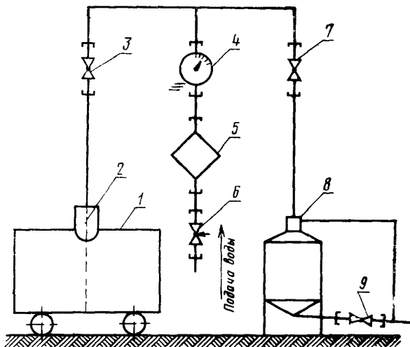
1—цистерна, 2—шланг, 3, 6, 7, 9—краны, 4—счетчик жидкости, 5—фильтр; 8—мерник
