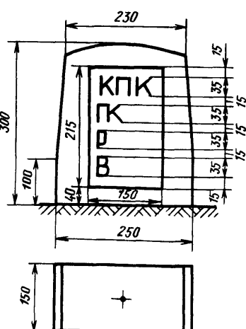
Середина переходной кривой
