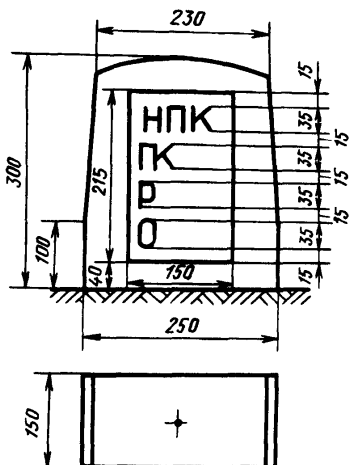
Начало переходной кривой
