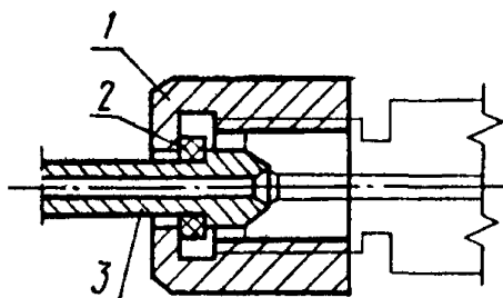
1 — накидная гайка, 2 — нажимная шайба, 3 — труба Черт 1
