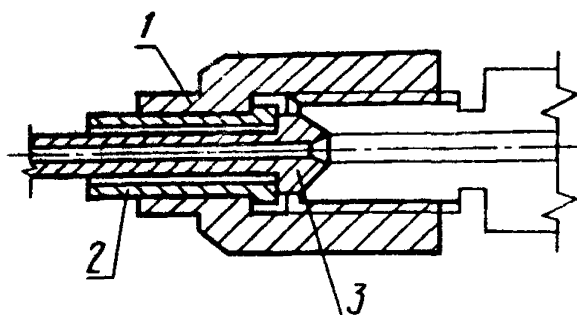
1 — накидная гайка, 2 — нажимная втулка, 3 — труба Черт 3
