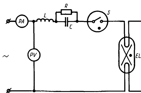
PA — амперметр; PV — вольтметр; EL — люминесцентная лампа; S — starter; L-C — индуктивно-емкостный балласт; R — резистор
