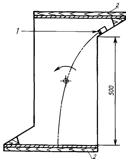
1 — starter; 2 — стальная плита толщиной 3 мм
