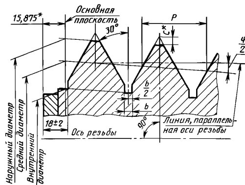
Профиль резьбы калибра-пробки
