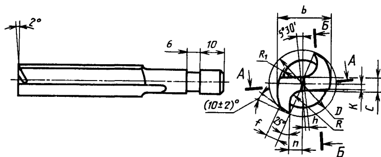
Исполнение фрез размером D=5 мм
