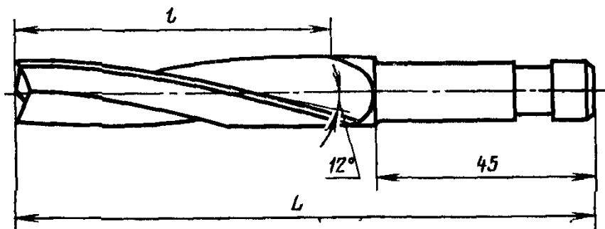
Вариант изготовления фрез типа 2 с винтовой канавкой
