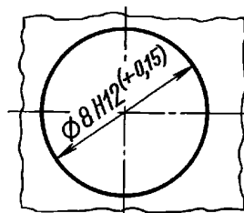
Разметка для крепления на панели
