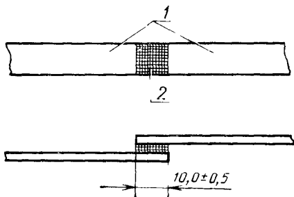
1—склеиваемый материал, 2—клеевое соединение
