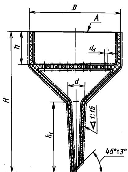
Кружка 2 ГОСТ 9147—80 Воронка Бюхнера
