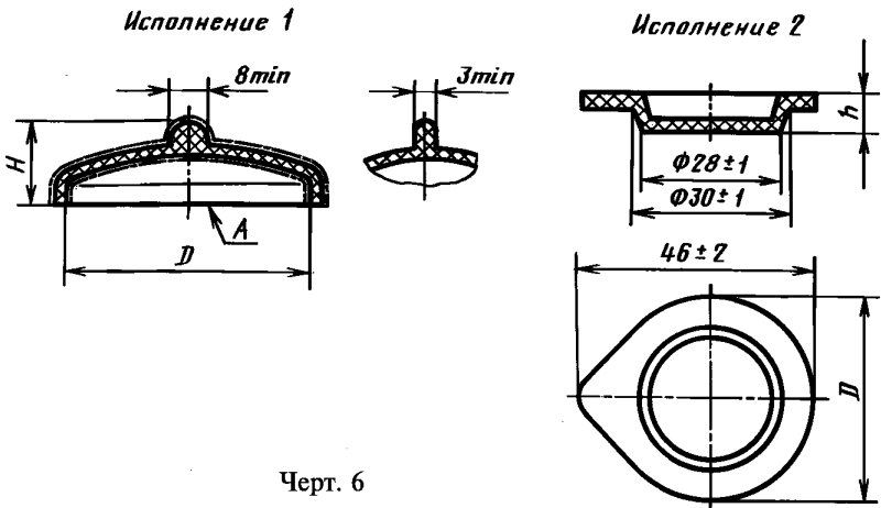
Крышки к тиглям
