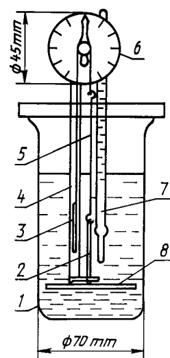
1 — стеклянный химический стакан; 2 — испытуемый образец; 3 — латунный груз; 4 — латунная трубка; 5 — крючок; 6 — круглая шкала; 7 — термометр; 8 — пруток
