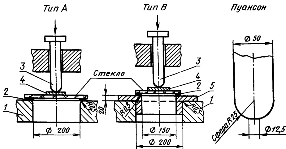
1 — плита матрицы; 2 — плоское кольцо; 3 — пуансон; 4 — прокладка; 5 — втулка Черт. 2
