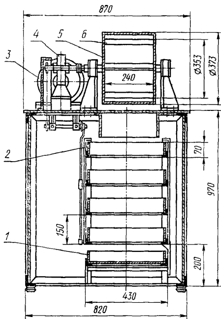
1—противень; 2—сито; 3—электромотор; 4—редуктор; 5—кожух барабана; 6—колосник.
