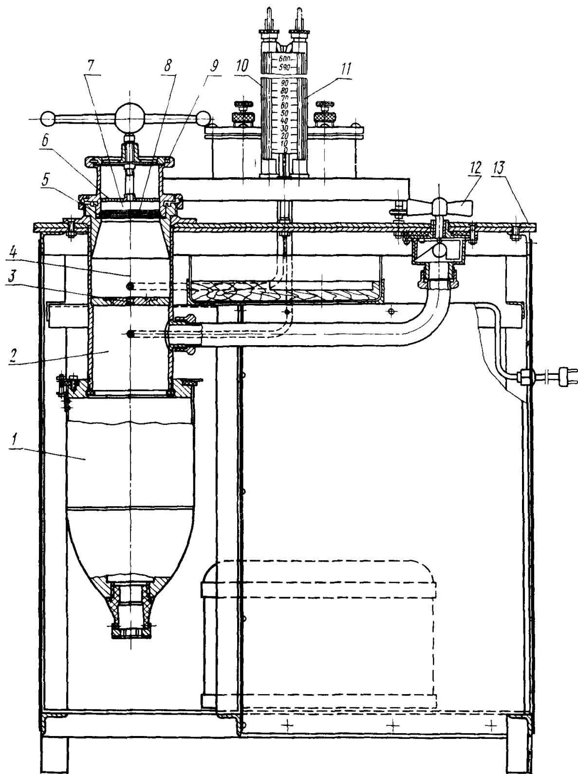
1—вентилятор; 2—камера, 3—диафрагма 4—камера 5—дно рабочей камеры; 6—крышка рабочей камеры, 7—рабочая камера, 8—фильтр, 9—запорное приспособление, 10—левый манометр 11—правый манометр, 12—дроссель, 13—стол
