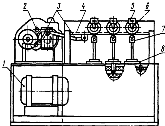
1 — электродвигатель; 2 — редуктор; 3 — кривошипно-шатунный механизм; 4 — зубчатая рейка; 5 — подвижный зажим; 6 — валик; 7 — подвесной зажим; 8 — груз
