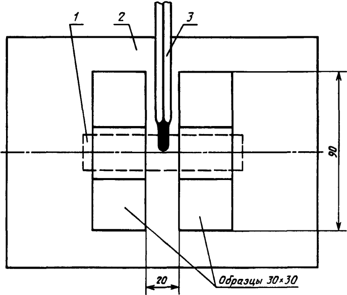
I — ртутно-кварцевый облучатель; 2 — лист асбестового картона; 3 — термометр
