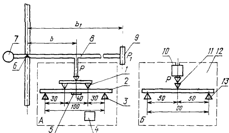
Схема установки для определения модуля упругости
