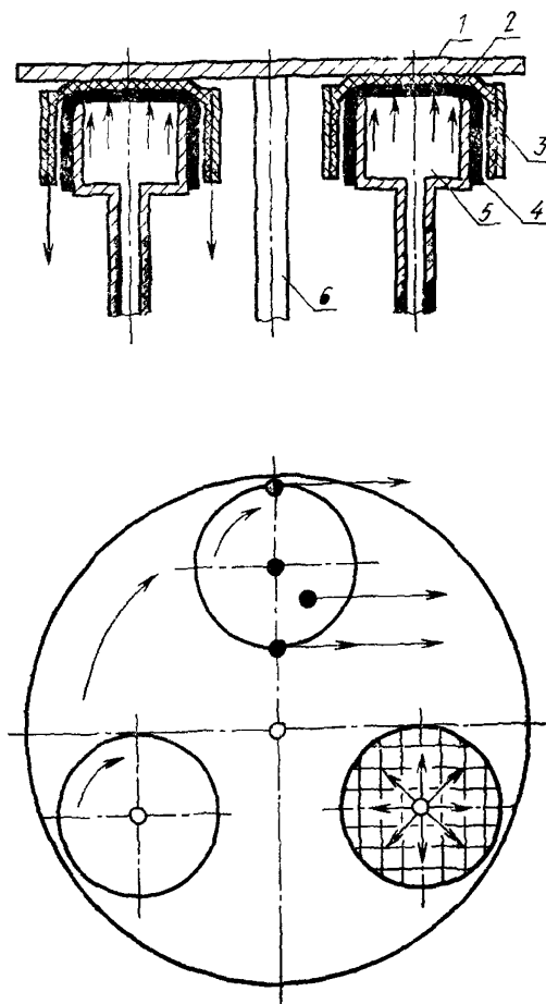
1 — истирающий диск; 2 — проба; 3 — обойма; 4 — мембрана; 5 — головка; 6 — ось
