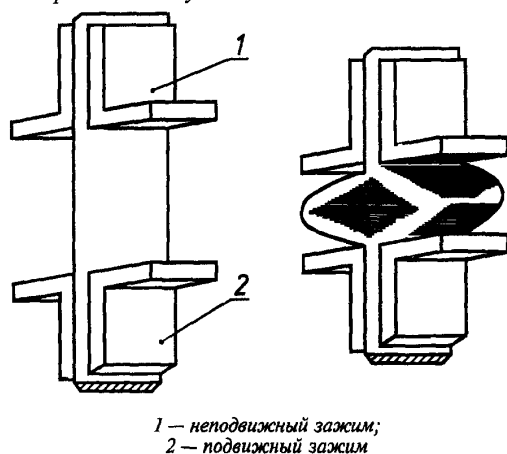
Рисунок 2 — Схема испытания материалов прибором типа МИРП
