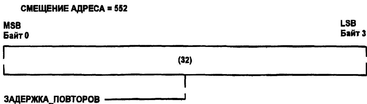
Рисунок 3—27 — Регистр ЗАДЕРЖКА_ПОВТОРОВ_ПРИ_ОШИБКЕ
