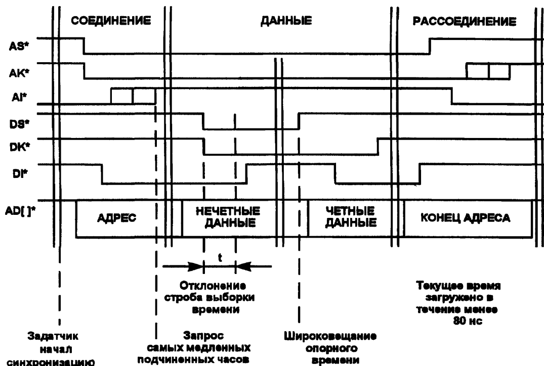
Рисунок 3—4 — Синхронизация часов
