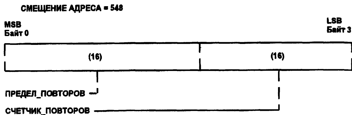
Рисунок 3—26 — Регистр СЧЕТЧИК_ПОВТОРОВ_ПРИ_ОШИБКЕ
