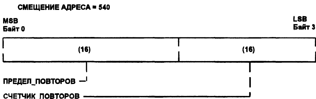
Рисунок 3—24 — Регистр СЧЕТЧИК_ПОВТОРОВ_ПРИ_ЗАНЯТОСТИ
