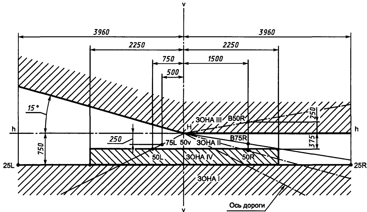
В — Фара для левостороннего движения (размеры в мм)
