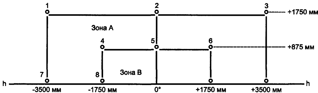
С — Точки измерения величин освещенности
