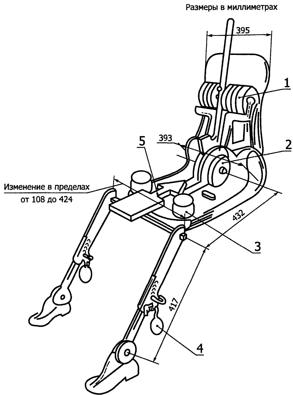
1 — спинные грузы; 2 — седалишные грузы; 3 — набедренные грузы; 4 — ножные грузы; 5 — направление и точка приложения нагрузки
