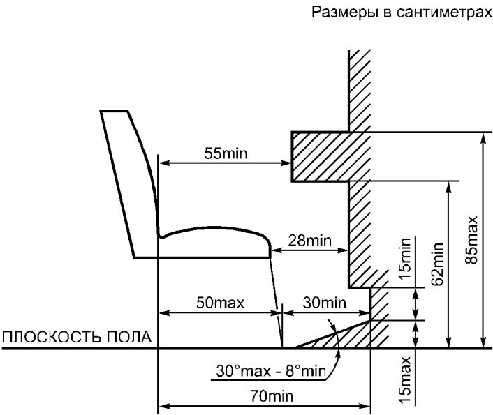
Рисунок 3.8 — Пространство для сидящих пассажиров (см. 5.7.8.5)
