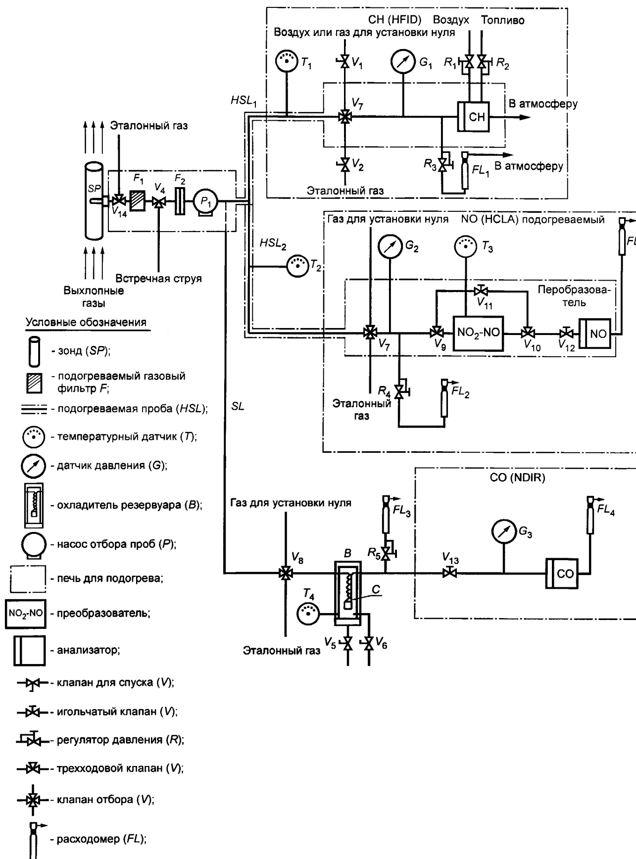
Рисунок 1 — Принципиальная схема системы анализа отработавших газов для измерения \text{CO} , \text{NO}_x и \text{CH} (анализ с помощью HCLA и подогреваемого трубопровода отбора проб)
