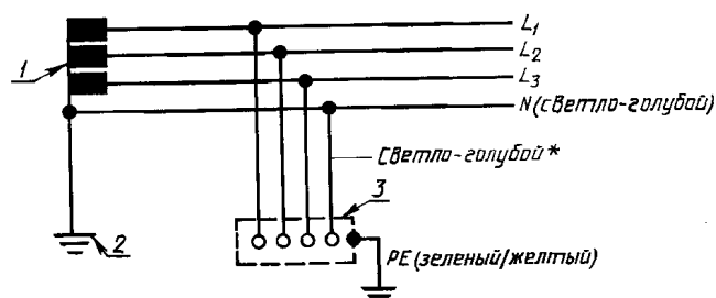
1 — точка заземления энергосистемы; 2 — земля; 3 — открытые проводящие части; L_1, L_2, L_3 — фазные проводники энергосистемы; PE — защитный проводник; N — нулевой проводник
