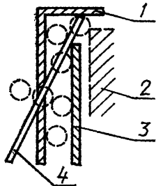
1 — оболочка; 2 — часть, находящаяся под напряжением; 3 — барьер; 4 — проволока или стержень.
