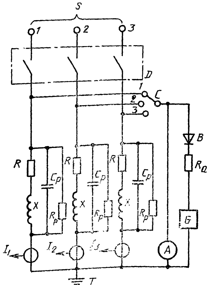
Схема способа регулировки цепи нагрузки
