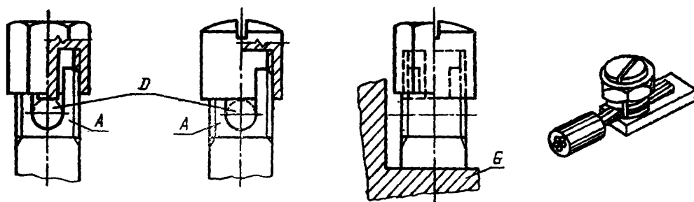
A — неподвижная часть; D — место для проводника; G — часть аппарата с полостью для вывода.
