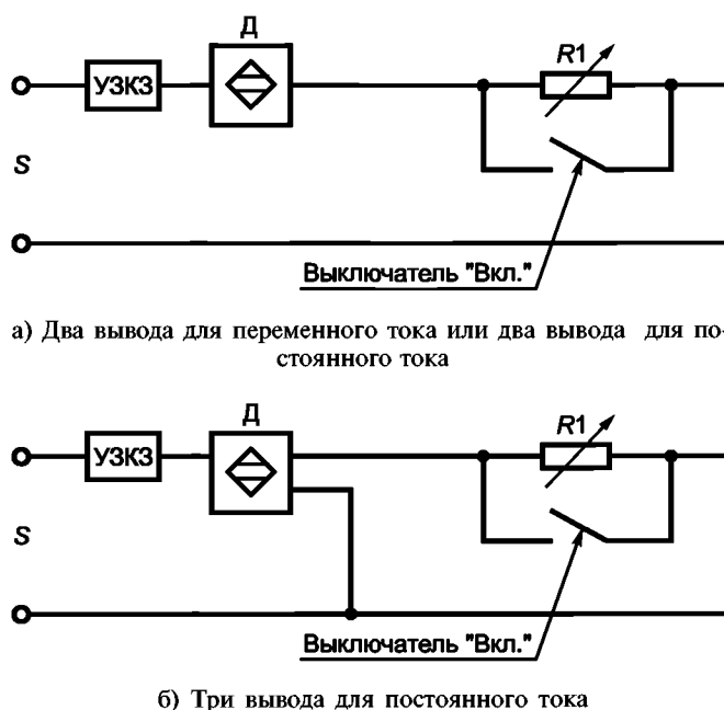
Рисунок 10 — Схема испытаний на короткое замыкание (см. 8.3.4.2)
