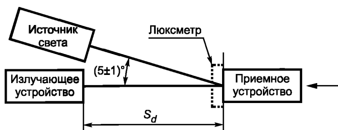
Рисунок 11a — Датчик типа Т, излучающее и приемное устройство
