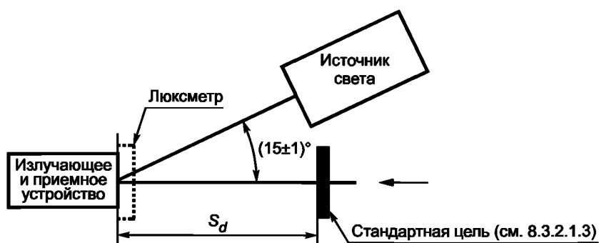
Рисунок 11c — Датчик типа D, излучающее и приемное устройство и стандартная цель
