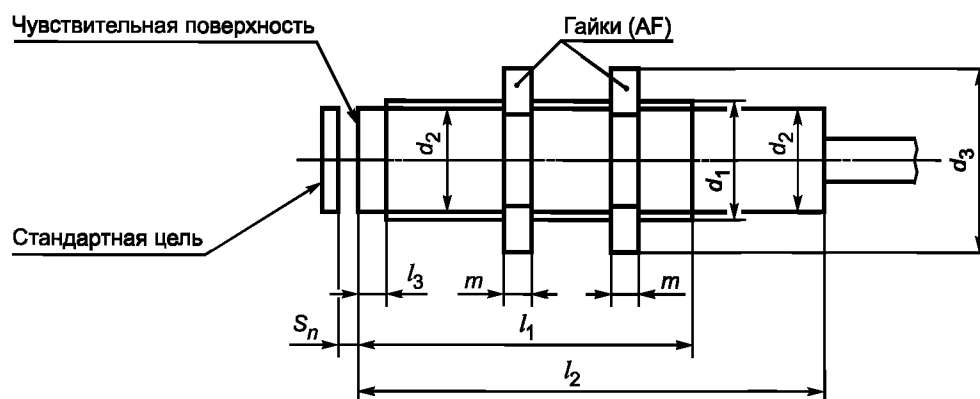
Рисунок А.1 (IА) — Габаритные размеры
