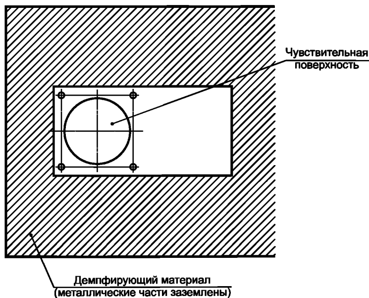
Рисунок A.2 (CD) — Установка (монтаж)
