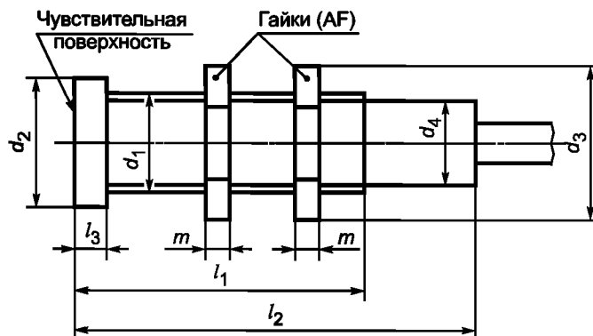
Рисунок A.1 (UA) — Габаритные размеры
