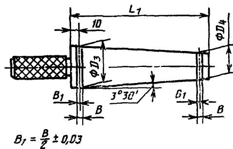
Калибр для патрона без закатанного торца
