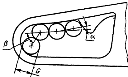
Клиренс за рычагом управления
