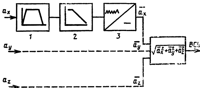
Взвешенное суммарное ускорение
