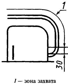
Рисунок 2 — Зона захвата передней рукоятки
