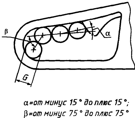
Рисунок 4 — Клиренс за рычагом управления
