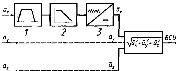
Рисунок В.1 — Взвешенное суммарное ускорение
