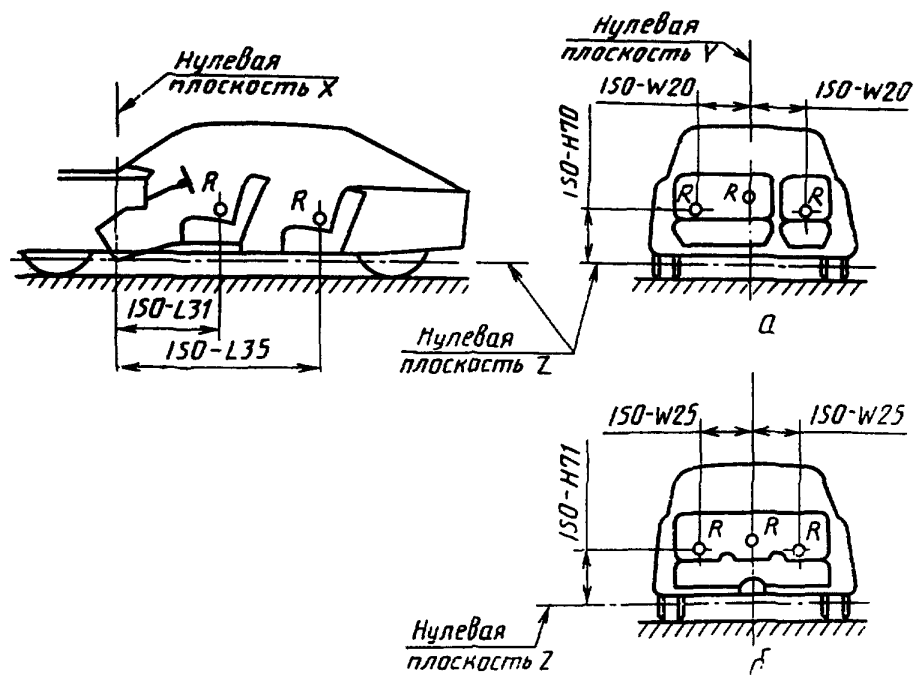
Черт. 4. Размеры, определяющие положение точек R
