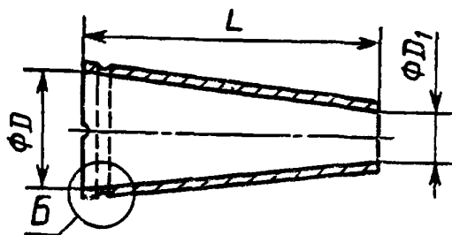
Конический патрон без закатки
