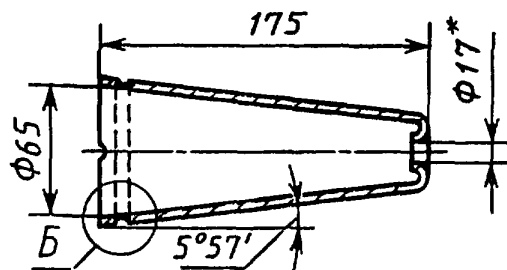
Конический патрон с закатанным торцом
