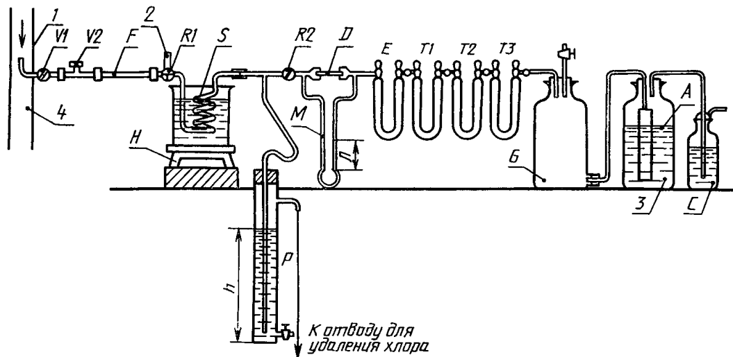
Схема аппарата для определения содержания воды в хлоре
