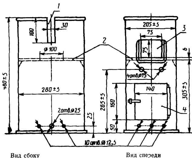
Вид сбоку Вид спереди 1 — щель; 2 — огнеупорная полка; 3 — слюдяное окошко; 4 — дверца
