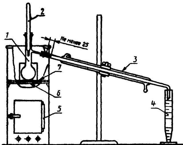
1 — дистилляционная колба (п. 4.1.1); 2 — термометр (п. 4.1.2); 3 — холодильник (п. 4.1.4); 4 — приемник (п. 4.1.3); 5 — защитный кожух (п. 4.1.5); 6 — огнеупорная прокладка (п. 4.1.6)
