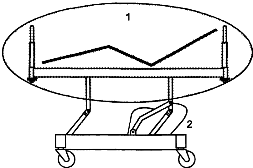
1 — область РАБОЧЕЙ ЧАСТИ; 2 — земля или выравнивание потенциалов Рисунок 111 — Зона РАБОЧИХ ЧАСТЕЙ и выравнивание потенциалов
