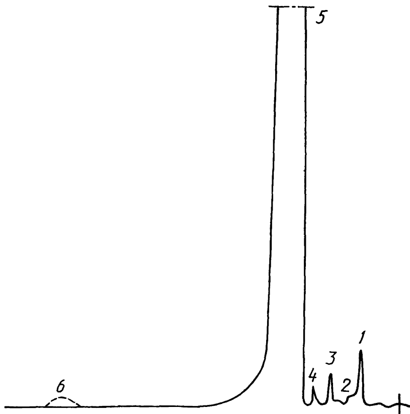
Типовая хроматограмма дифторхлорметана
